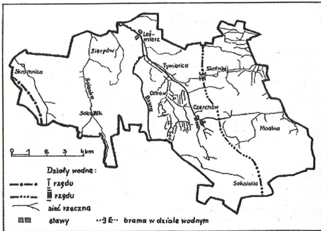
Rys. 9. Wody
