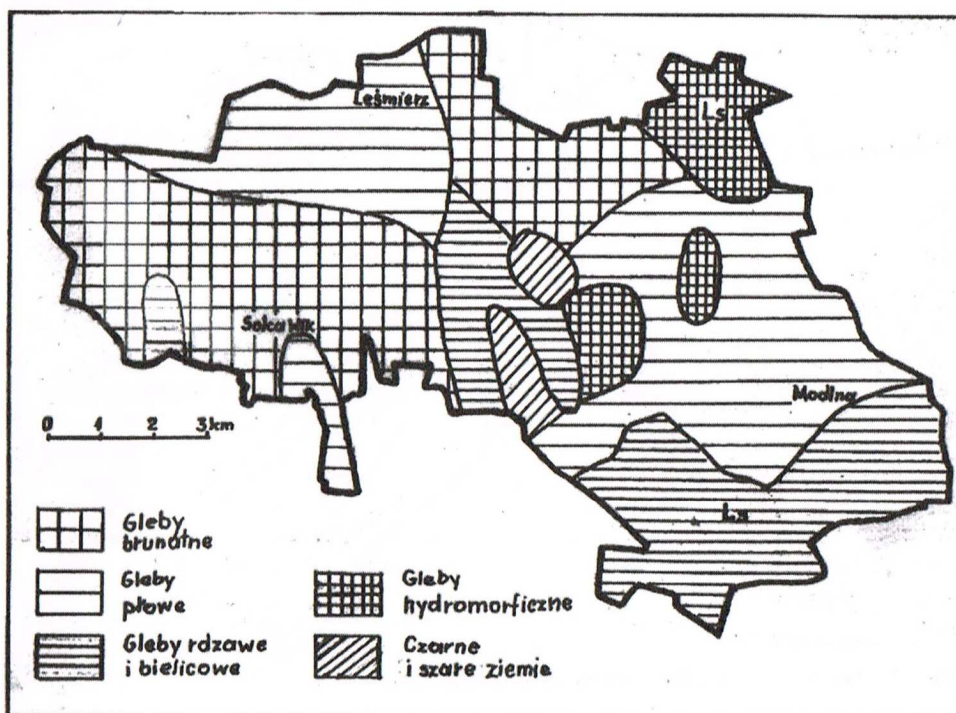
Rys. 10. Gleby
