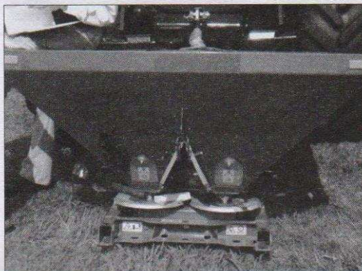
Rzysiwacz, który wzbudził wątpliwości dotyczące bezpieczeństwa (brak osłony tarcz wysiewających).
